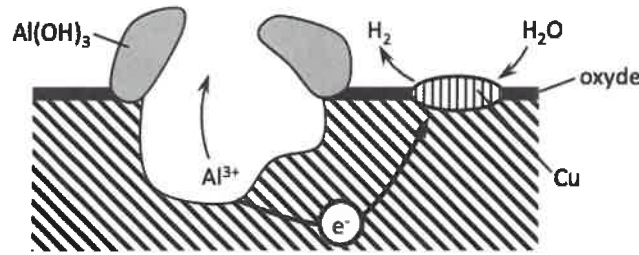
Figure 11 Phénomène de corrosion par piqure (d'après Techniques de l'ingénieur , Corrosion des alliages d'aluminium, Reboul M.)
