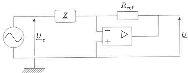
Figure 2 Schéma d'un impédancemètre
