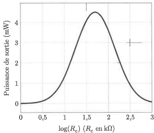
(a) Puissance de sortie
