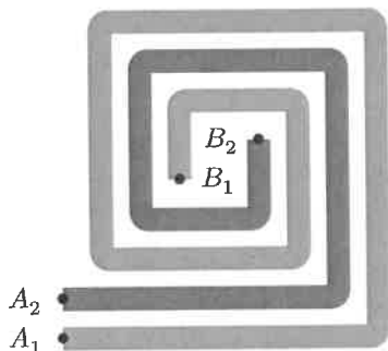
(a) Enroulements primaire et secondaire
