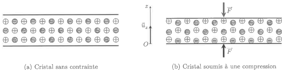
Figure 7 Cristal piézoélectrique
