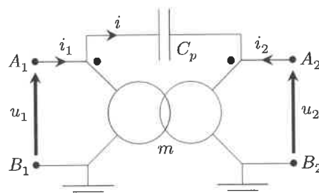
(b) Modélisation du transformateur complet
