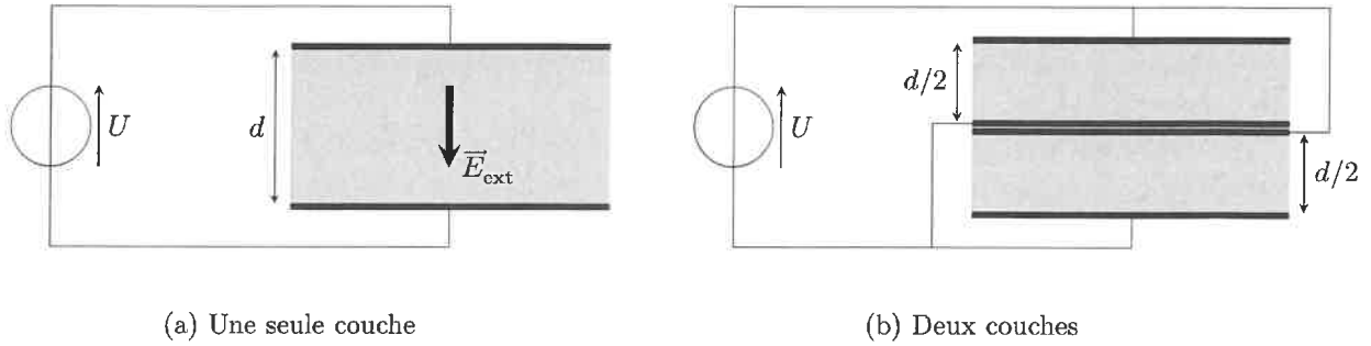
Figure 8 Matériau piézoélectrique placé dans un champ électrique
