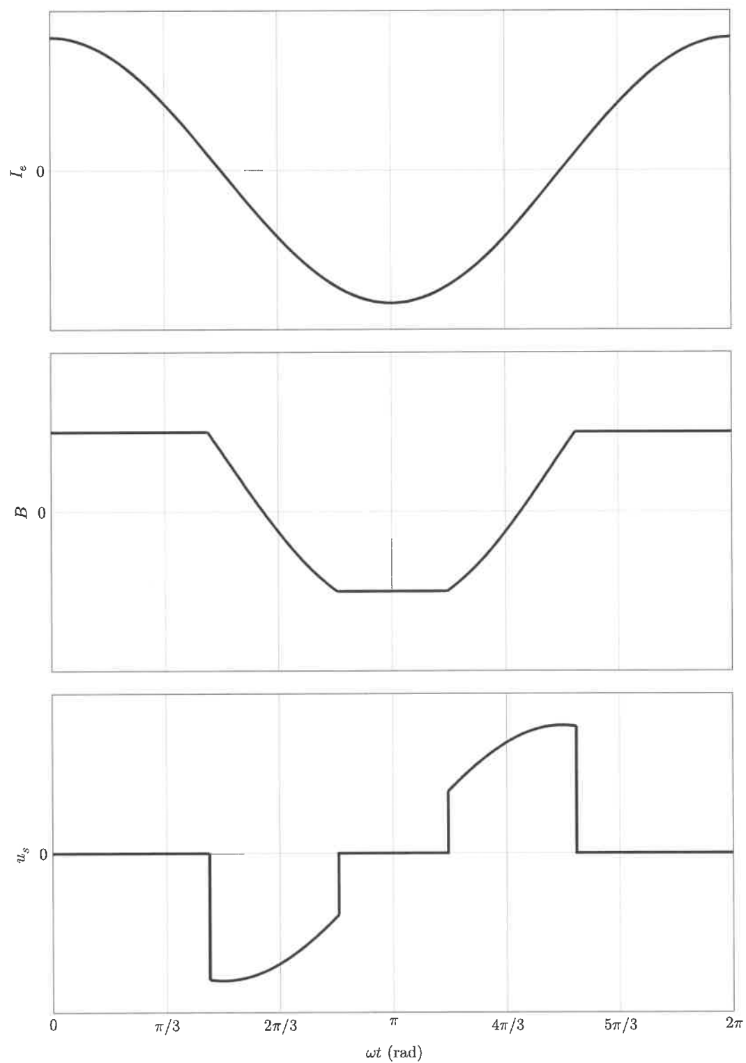
Figure C Graphes en présence d'un champ magnétique extérieur
