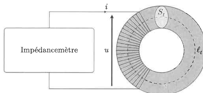
Figure 6 Tore de mesure d'impédance
