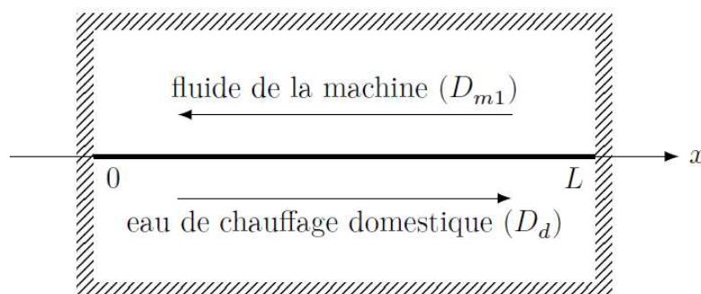
Figure 11 Schéma du condenseur
