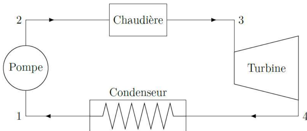
Figure 9 Schéma d'une centrale à vapeur
