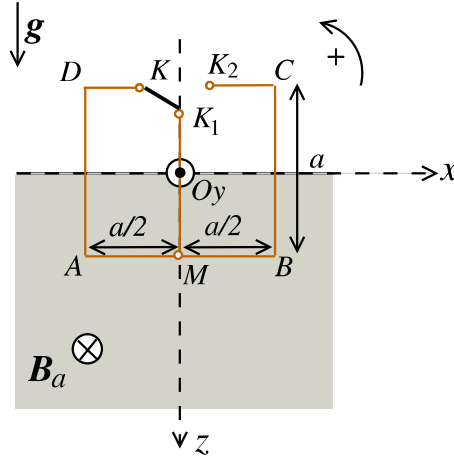
FIG. 4 – Cadre m  tallique pr  sentant un interrupteur K
