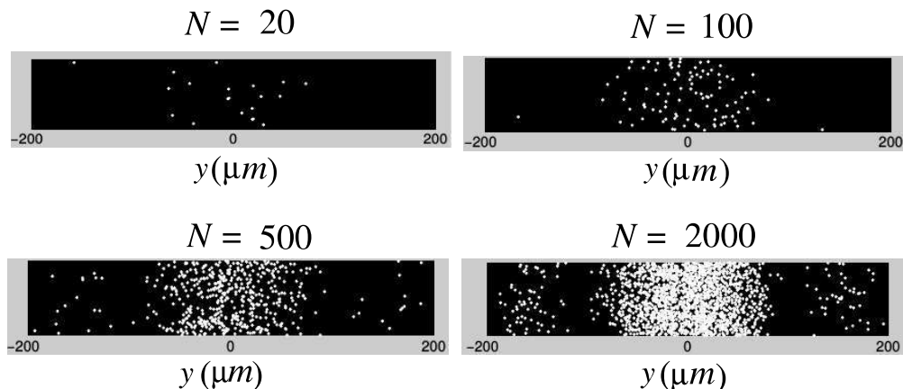
FIG. 6 – Distribution des impacts des neutrons sur l'écran
